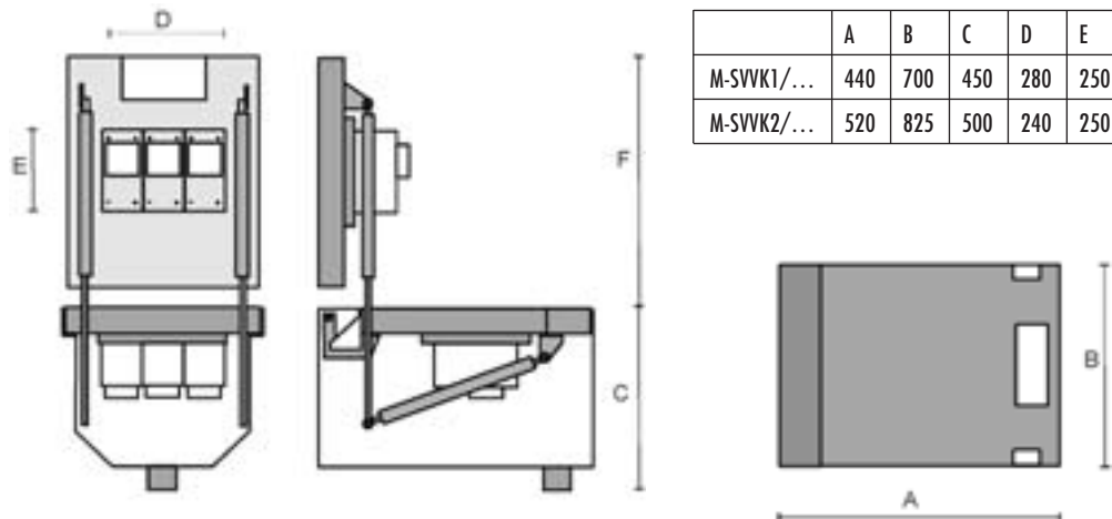
M-SVVK1/2D bestückt mit 2x Druckluftschnellkupplung
